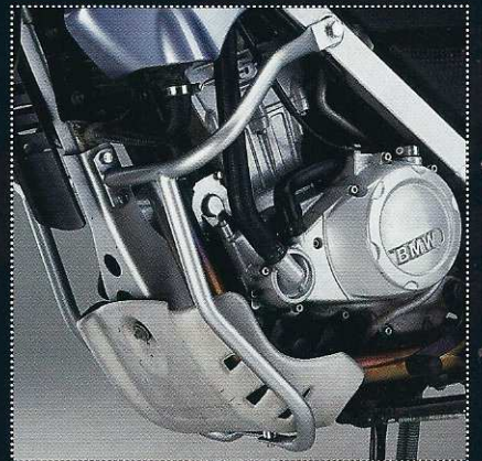
Enduro-Schutzbügel „ES“ Off-Road Protection Guard „ES“
